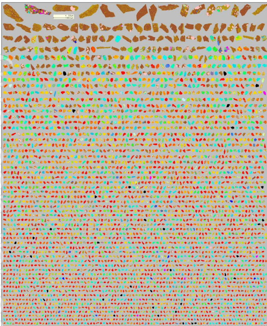
FM05: Leucoxene
