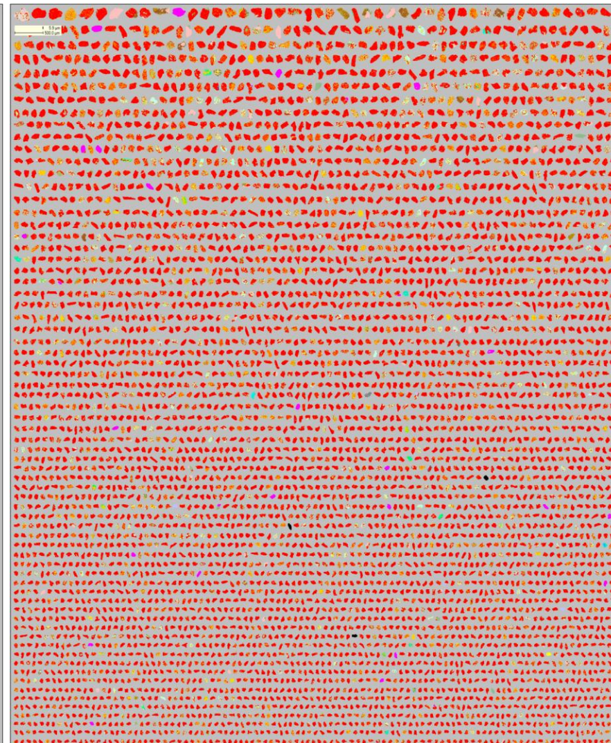
FM06: Rutile
