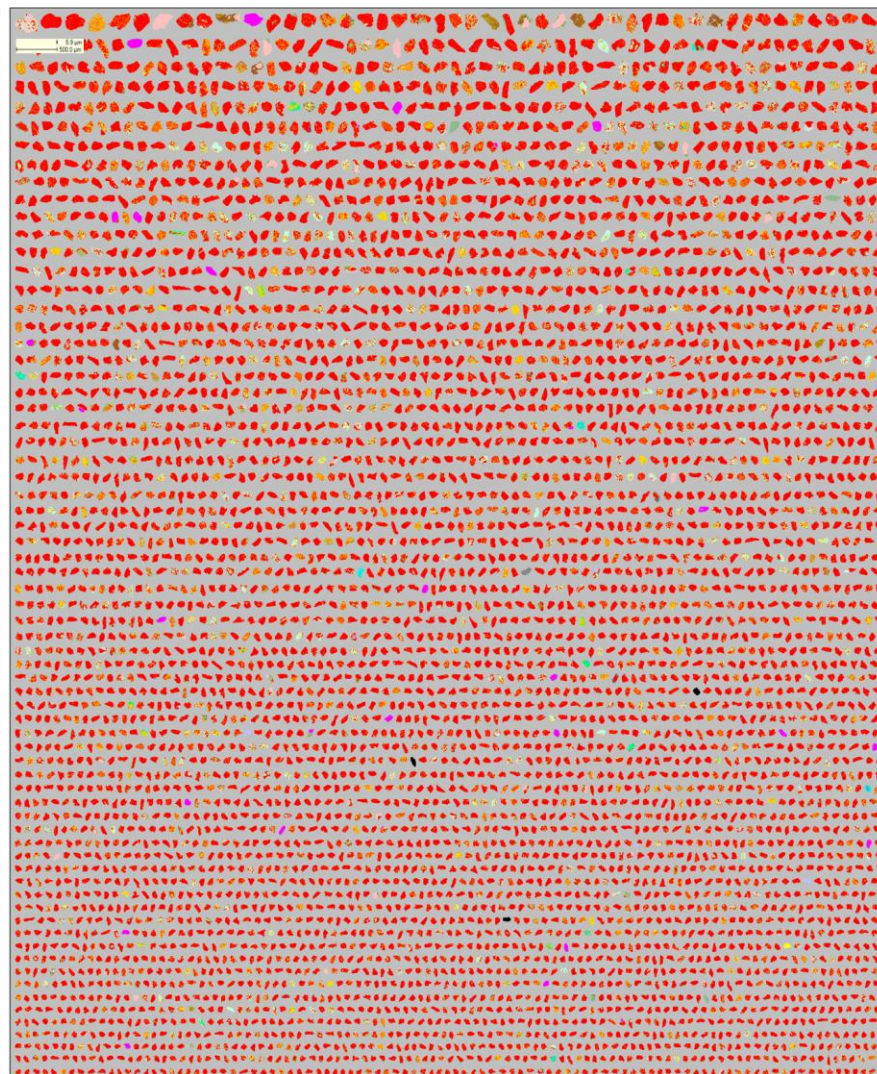
FM06: Rutile
