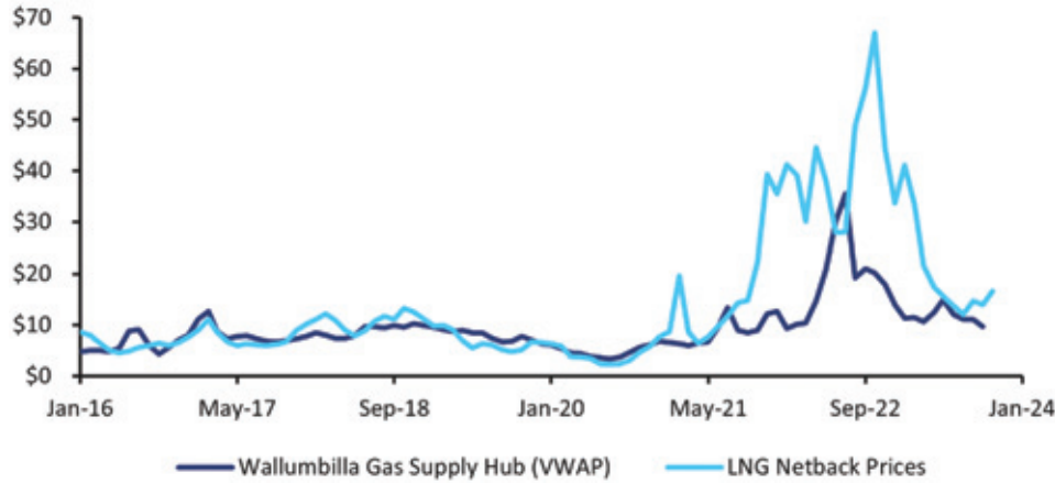
LNG Netback and Wallumbilla Prices (A$/GJ)
